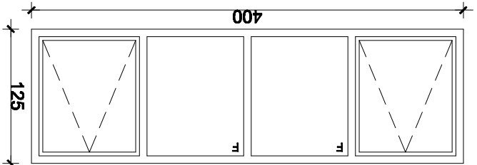
st.G/1.d-prozor vel.400x125cm- dva mehanizma za visoko otvaranje
